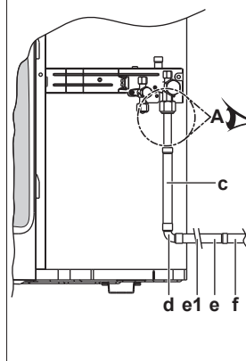
Вариант 3: подсоединение сбоку
